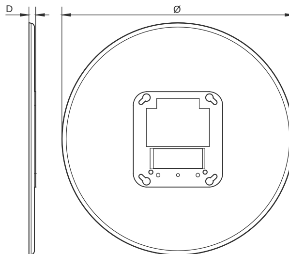
Figura 2: Dimensões
