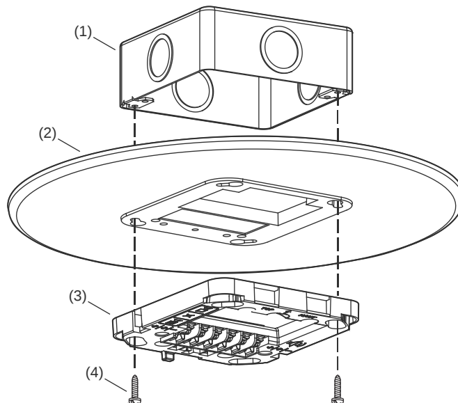
Figura 1: Montagem em uma caixa elétrica de uma posição
