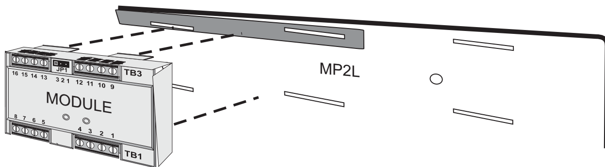
Figure 2, Montage d'un module sur la MP2L
