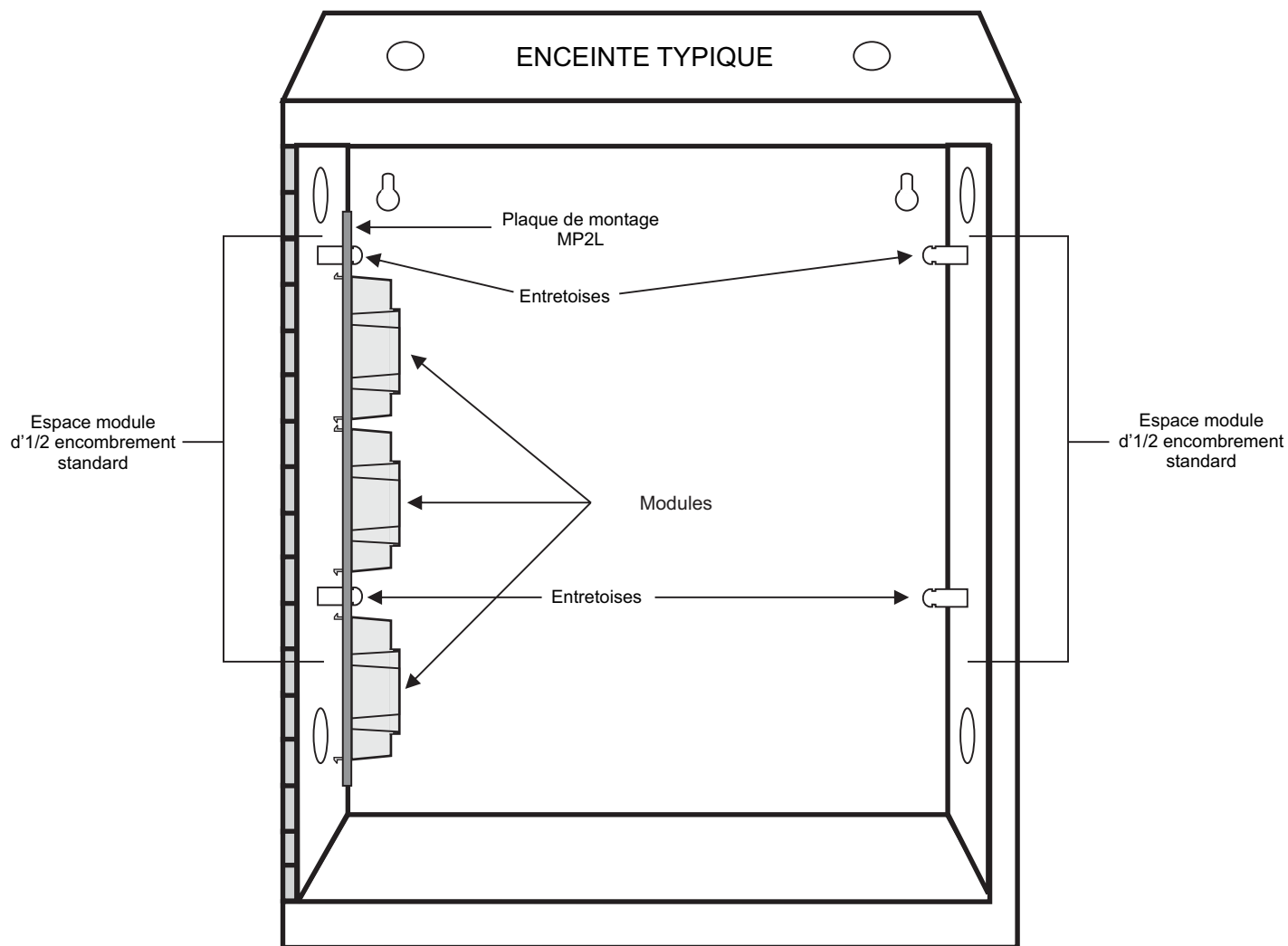
Figure 3, Montage de la MP2L à l'enceinte Espace module égal à \frac{1}{2} encombrement standard
