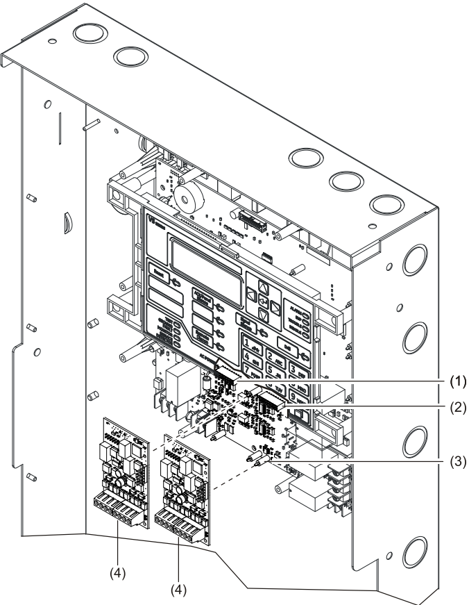
Figura 2: Instalação do V-SLC2-2 em um painel VS4
