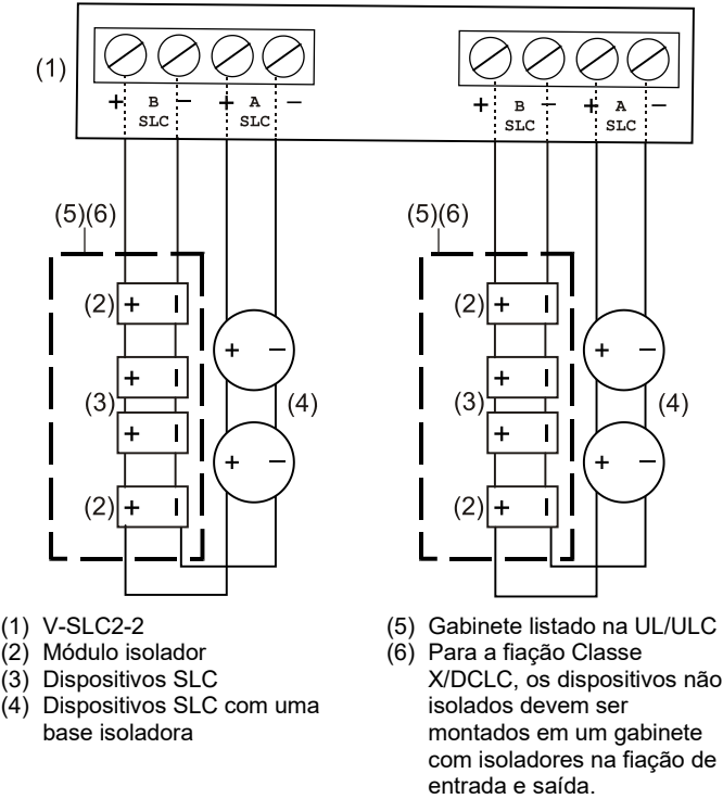
Figura 6: Fiação Classe X/DCLC [2]
