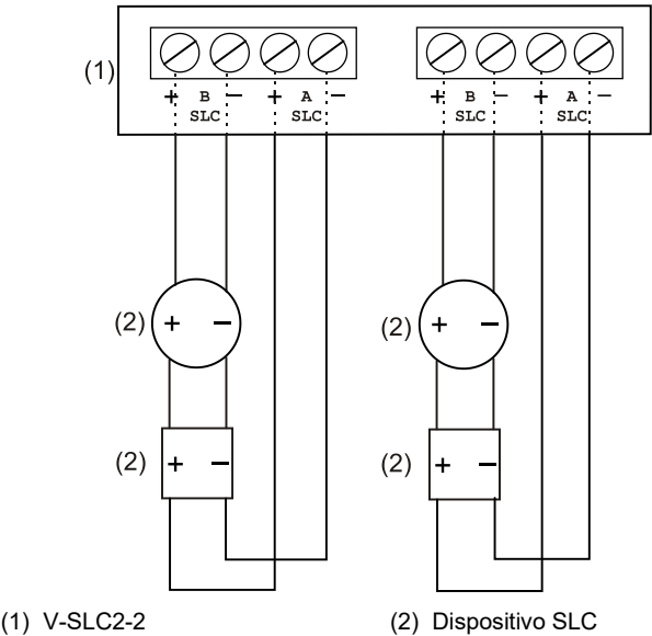
Figura 6: Fiação Classe X/DCLC [2]
