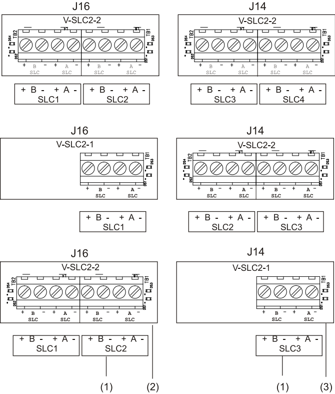
Figura 3: Configurações de número de painel SLC para o painel VS4
