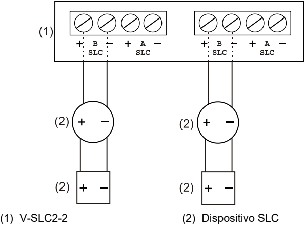
Figura 4: Fiação Classe B/DCLB
