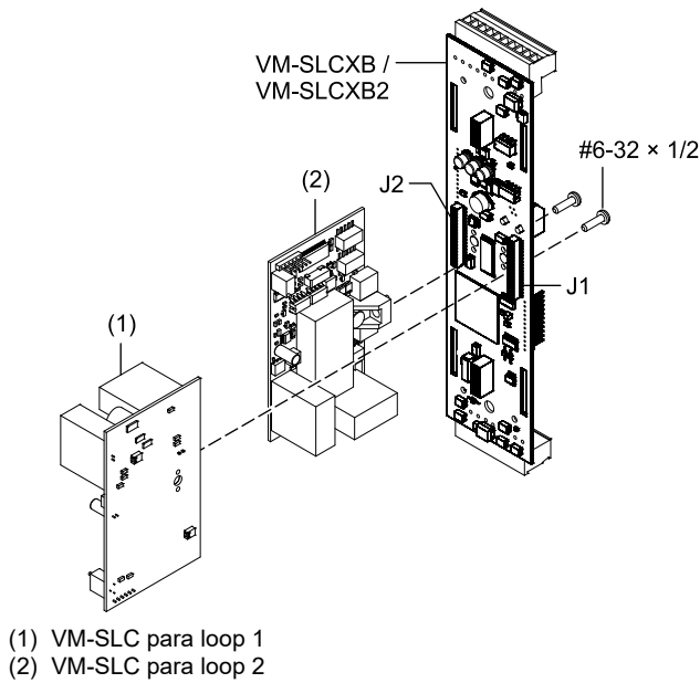
Figura 2: Instalando o VM-SLC em um módulo de controlador de loop VM-SLCXB / VM-SLCXB2
