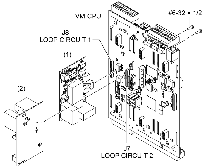
Figura 1: Instalando o VM-SLC em uma placa maior VM-CPU
