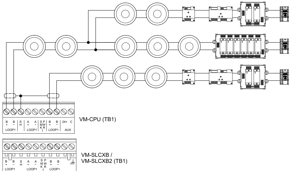
Figura 3: Ligação de Classe B
