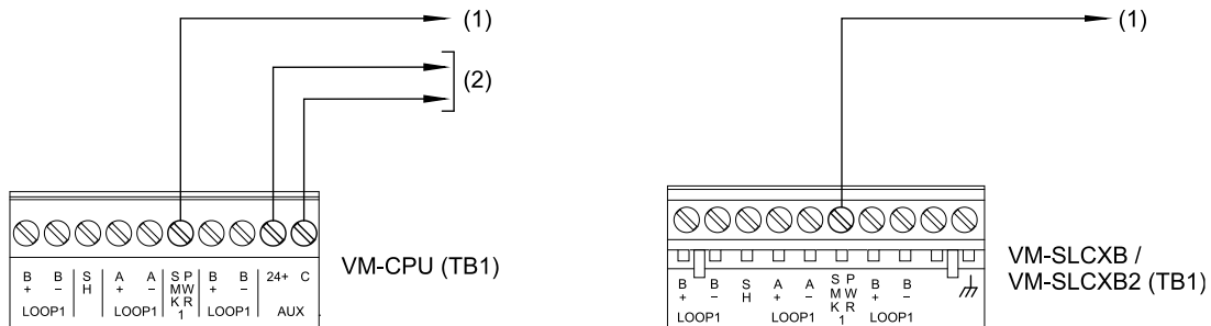
Figura 5: Ligação energia de fumaça e AUX
